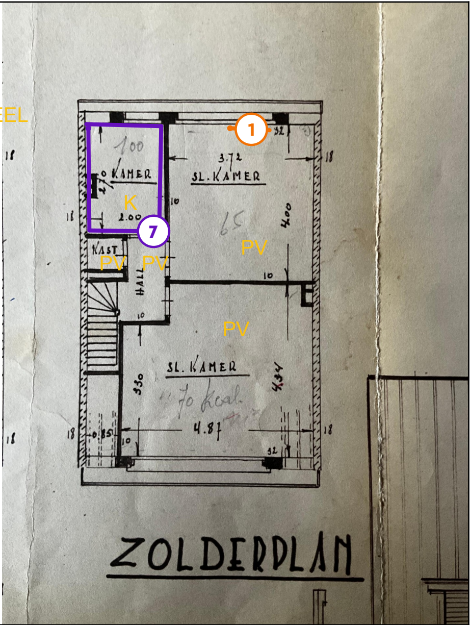
Legende van plan 1.4: plan 2e verdieping
