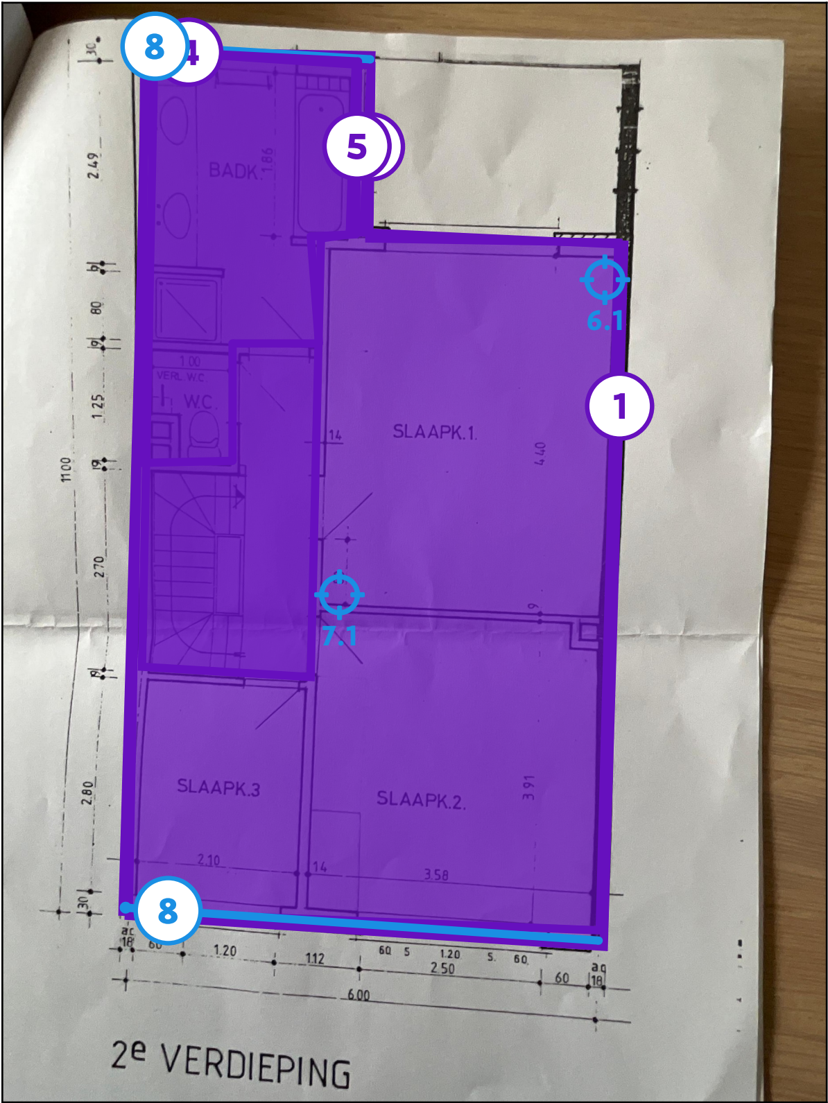
Legende van plan 1.4: Niveau +2
