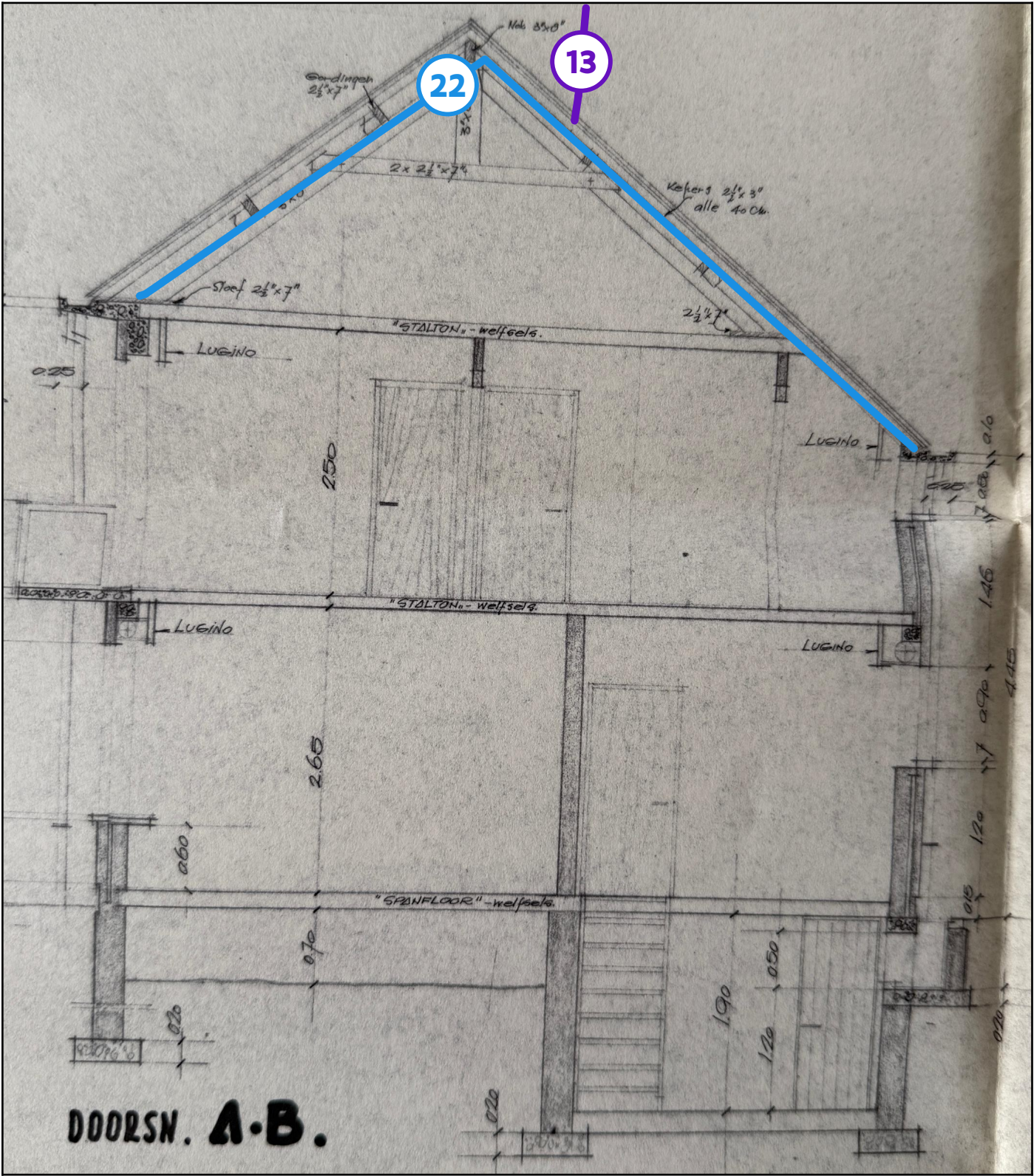
Legende van plan 1.4: snede
