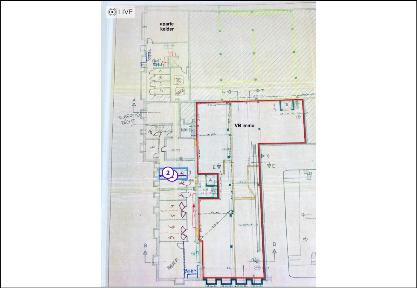
Legende van plan 1.4: kelder -1
